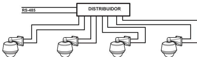
Esquema em estrela de interligação RS485
