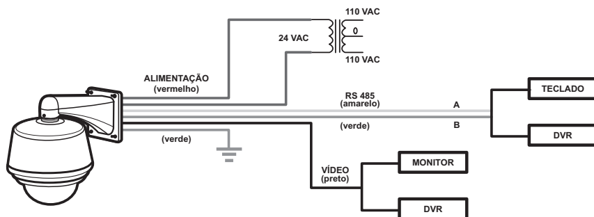
Esquema básico
