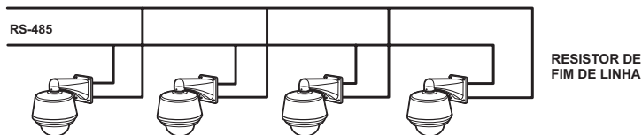
Esquema em linha de interligação RS485
