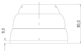
Visão lateral
