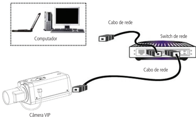
Conexão através de switch
