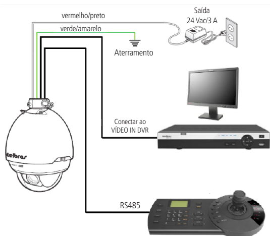
Esquema básico de controle SD
