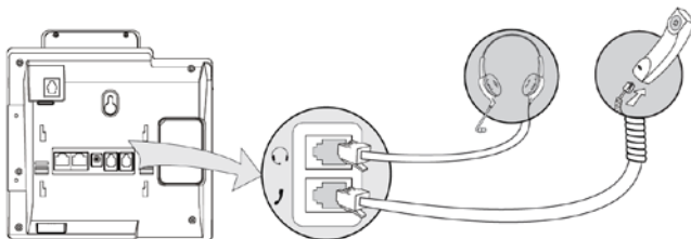
Instalação Headset
