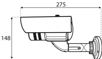
Vista lateral (sem o extensor)
