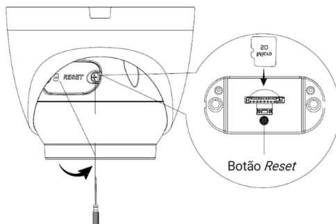
Acesso ao botão de Reset e SD Card das VIPW 1220 D FC e VIPW 1220 D FC PLUS
