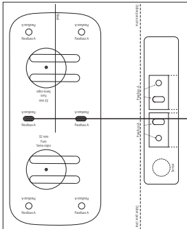
Abertura para fora Lado direito
