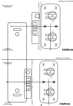
1× gabarito de furação
