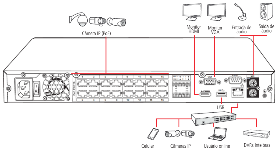
Exemplo de conexão NVD 3316 P
