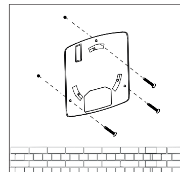
Fixando bracket na parede
