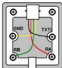
Tomada para instalação do TI 830i
