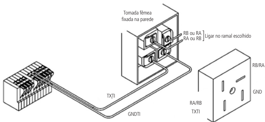
Instalação com tomada fêmea
