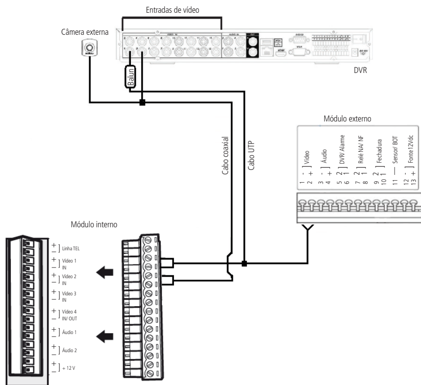
Ligação de vídeo paralelo com DVR
