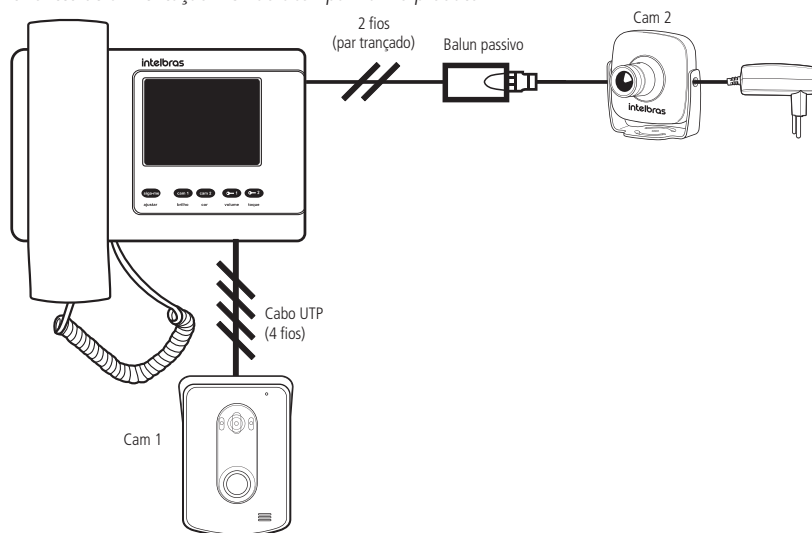
Instalação com câmera extra
