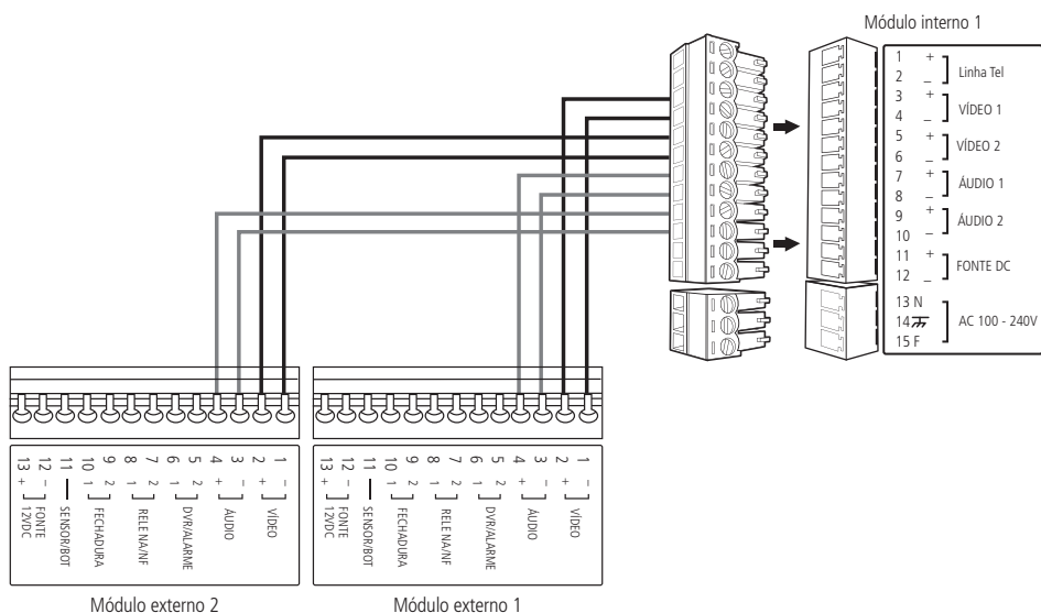
Conexão com 1 módulo interno e 2 módulos externos
