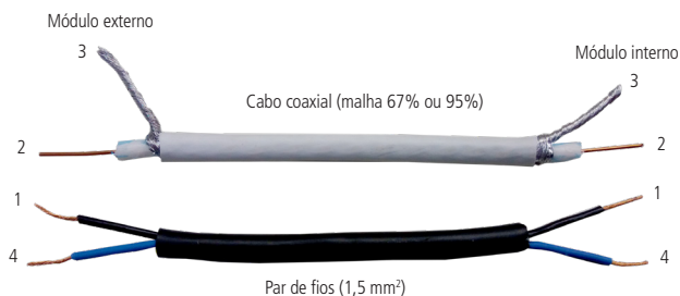
Instalação com cabo coaxial até 100 metros
