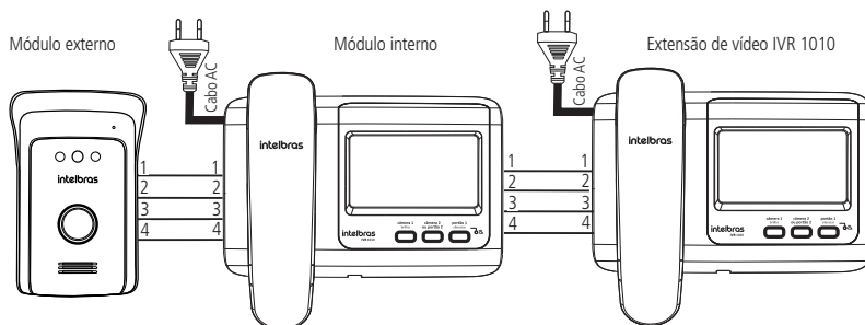
Instalação da extensão de vídeo com o IVR 1010
