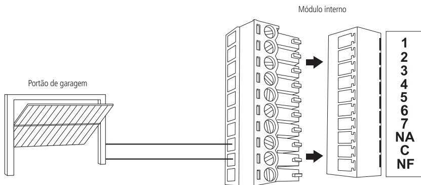
Instalação de portão de garagem
