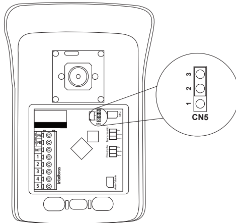
Ajuste do jumper CN5
