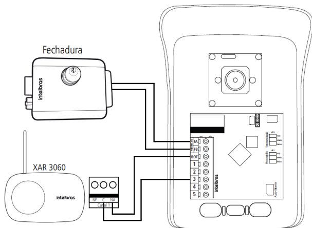
Integração com XAR 3060
