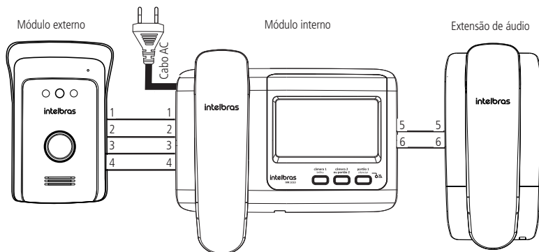
Instalação de extensão de áudio
