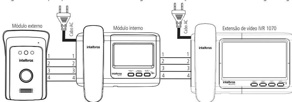
Instalação da extensão de vídeo com o IVR 1070
