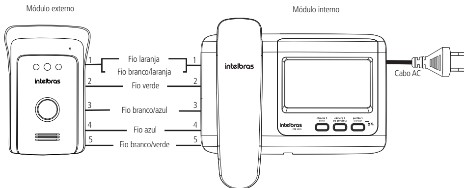
Instalação até 100 metros
