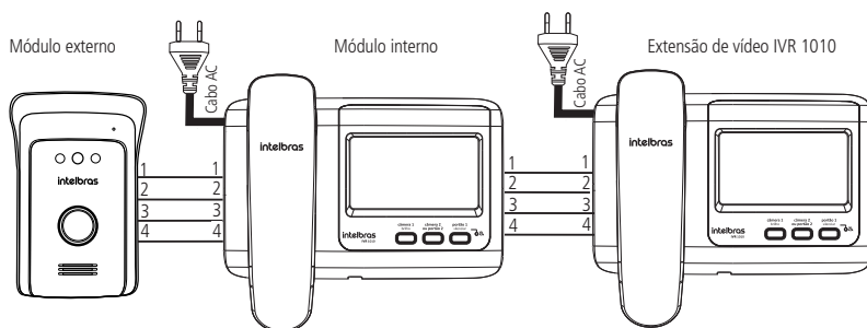
Instalação da extensão de vídeo com o IVR 1010
