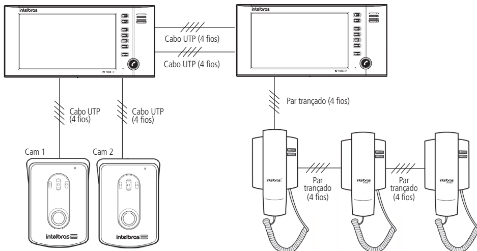
Instalação com 2 kits IV 7010 HF e 3 extensões de áudio
