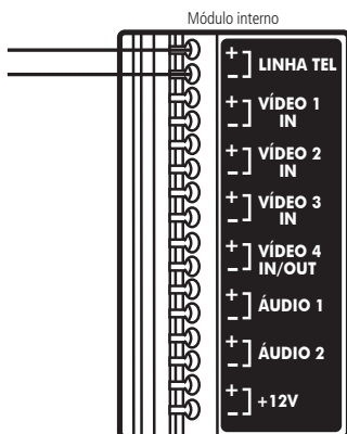
Instalação da linha telefônica
