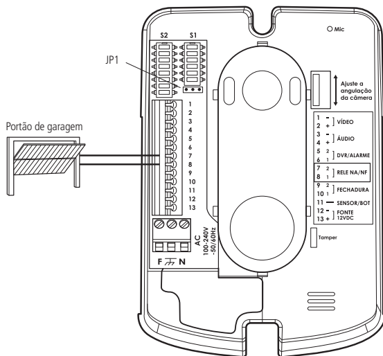
Instalação da fechadura 2
