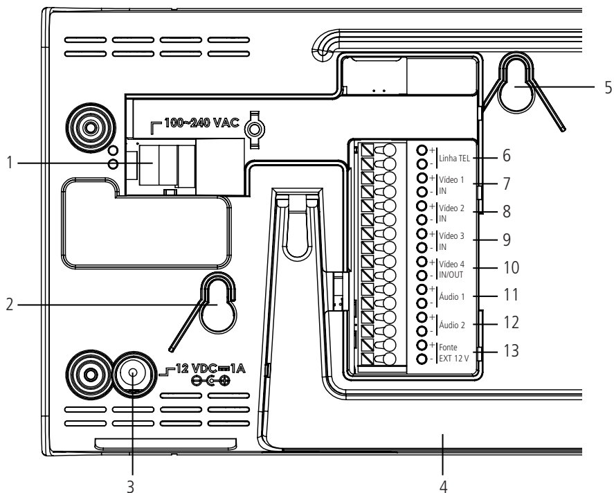
Vista posterior
