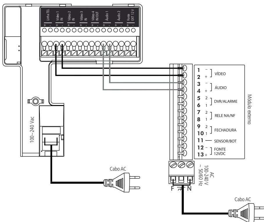
Instalação básica em AC
