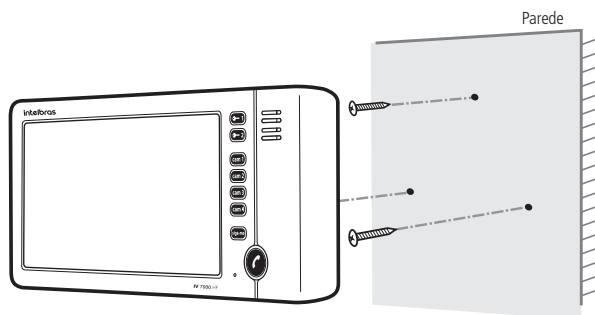
Encaixe nos parafusos
