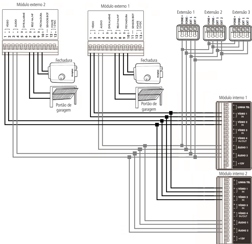
Conexão com 2 kit IV 7010 HF e 3 extensões de áudio
