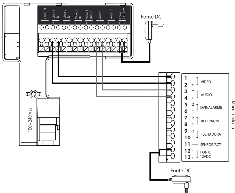
Instalação básica com fonte DC
