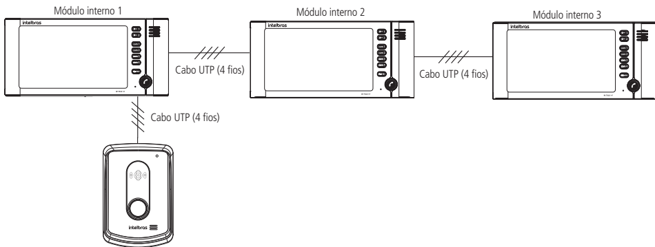
Instalação com 3 módulos internos e 1 módulo externo
