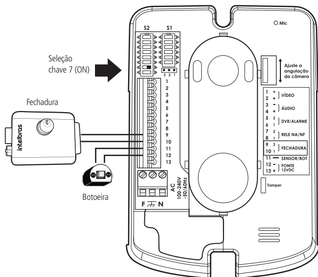
Instalação de fechadura com botoeira
