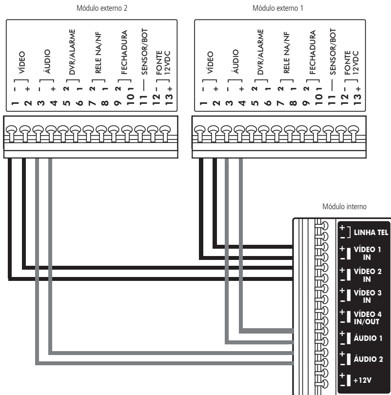
Conexão com 1 módulo interno e 2 módulos externos
