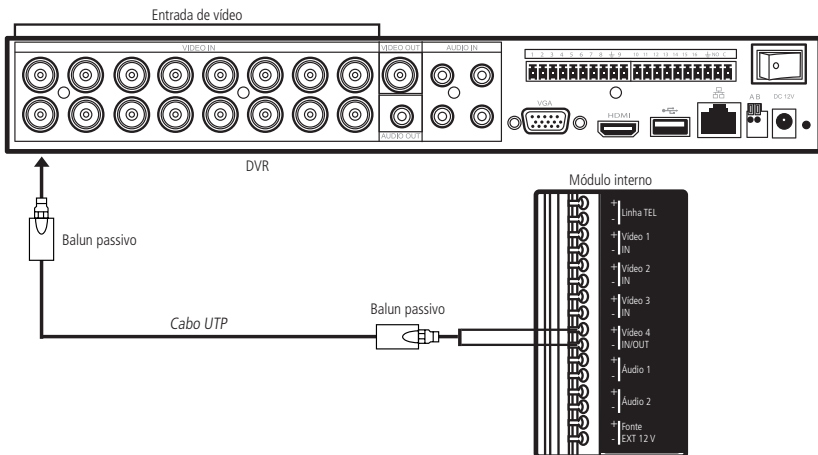
Gravar imagens do videoporteiro no DVR (Cabo UTP)
