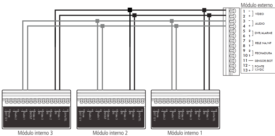
Conexão com 3 módulos internos e 1 módulo externo
