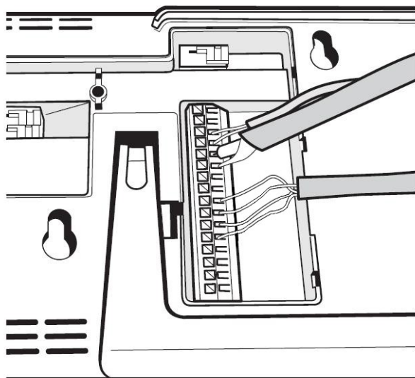
Conexão dos cabos
