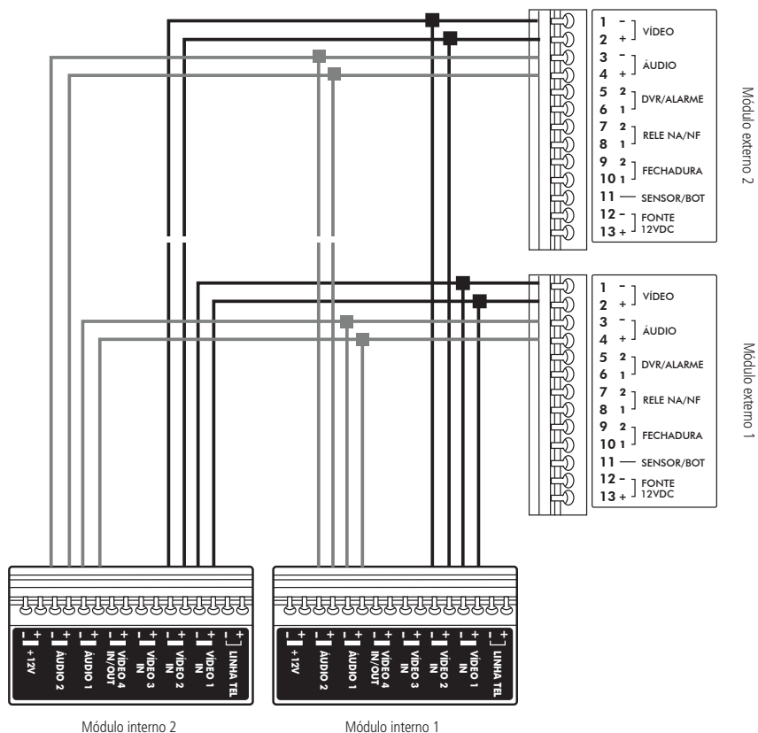
Conexão 2 módulos internos e 2 módulos externos
