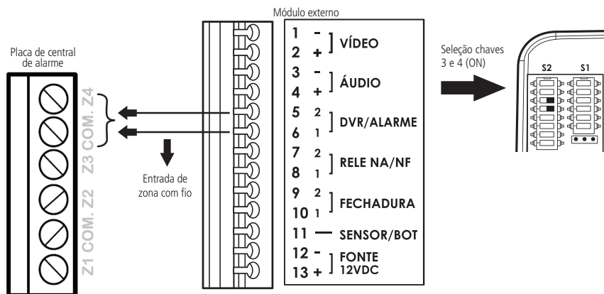
Integração com alarme
