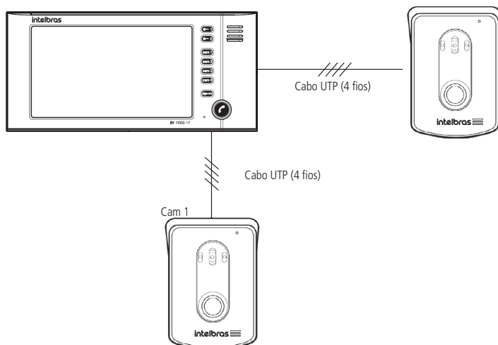
Instalação com 1 módulo interno e 2 módulos externos
