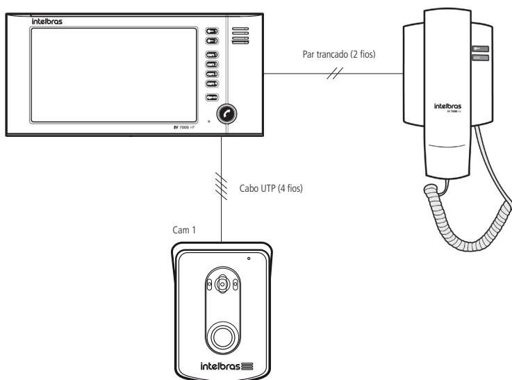
Instalação do IV 7010 HF e 1 extensão de áudio
