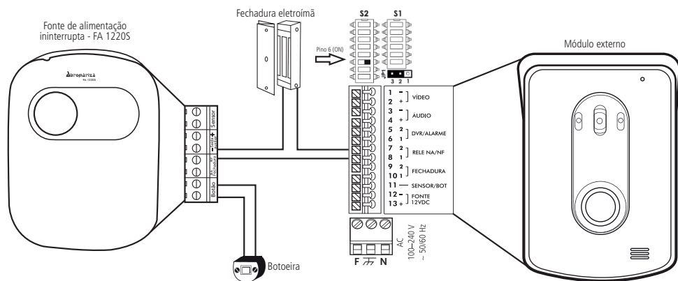
Instalação de fechadura-eletrôimã
