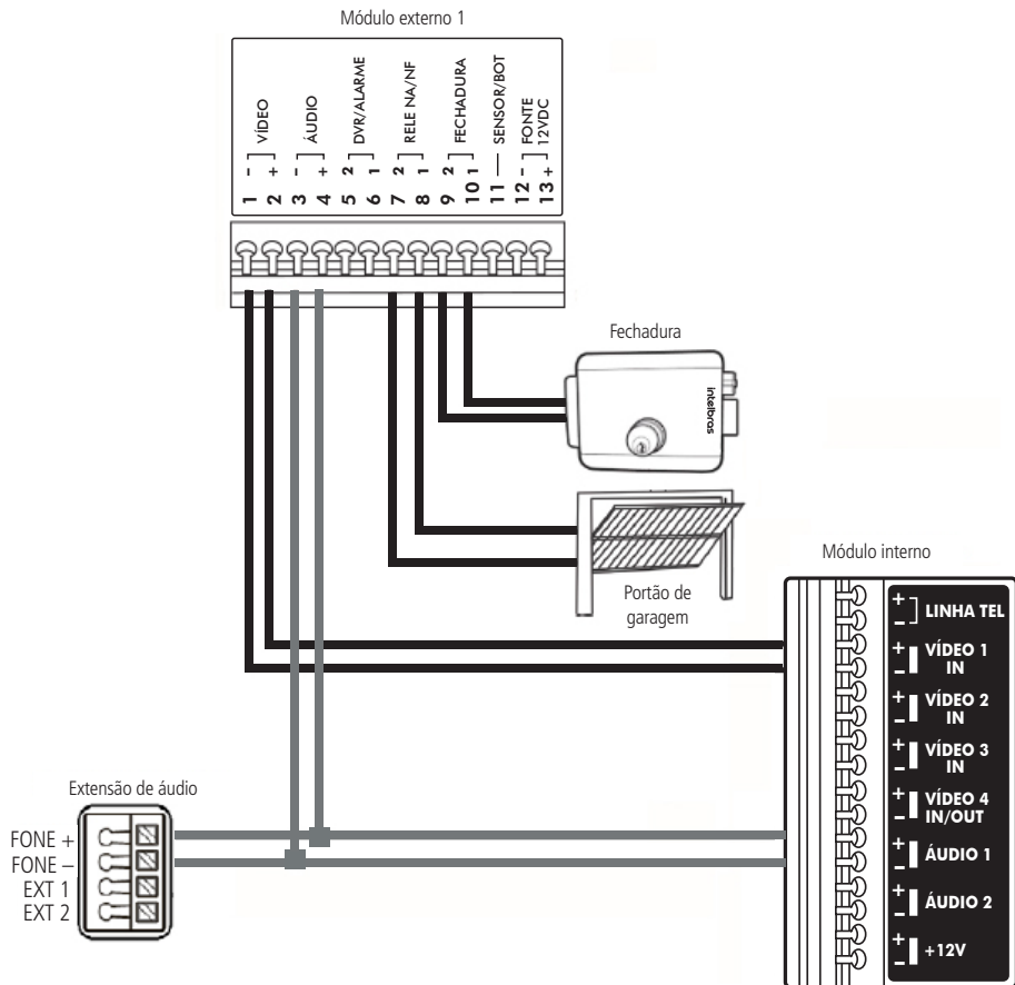
Conexão com o kit IV 7010 HF e 1 extensão de áudio
