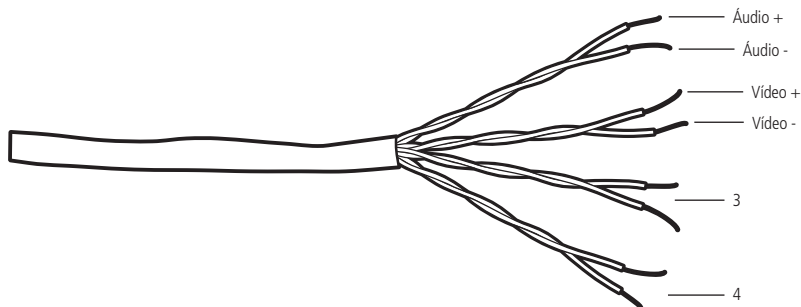
Instalação até 100 metros com cabo UTP
