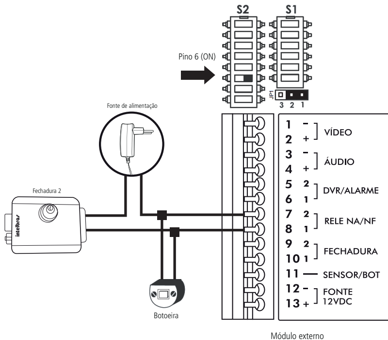
Instalação de segunda fechadura elétrica 2
