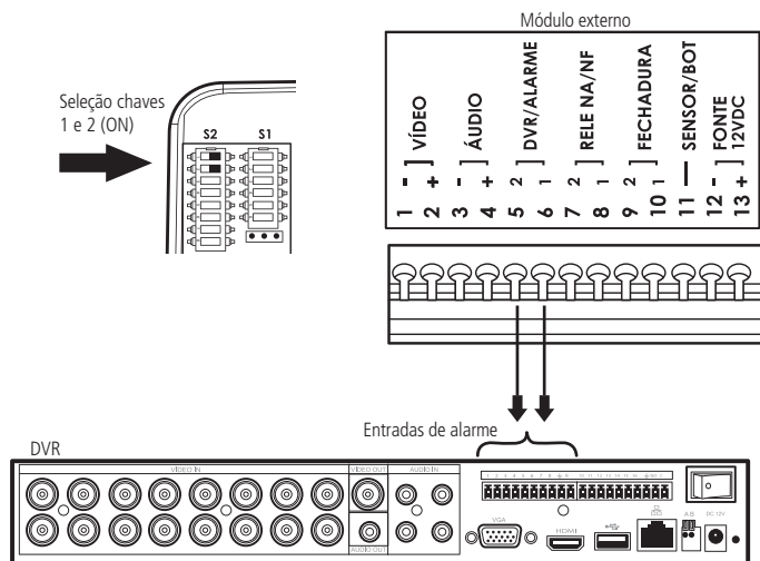
Integração com DVR - Saída DVR/ALARME
