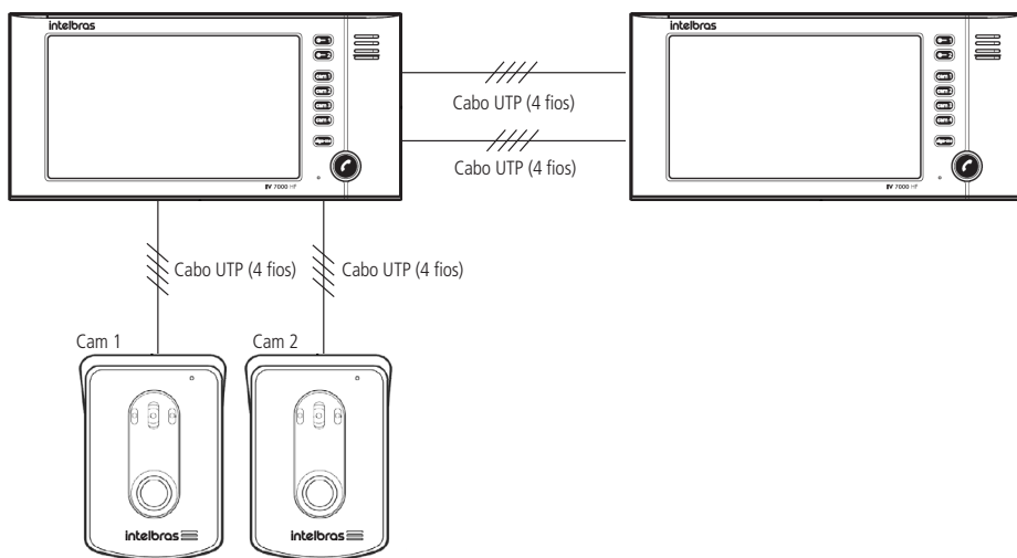
Instalação com 2 módulos internos e 2 módulos externos
