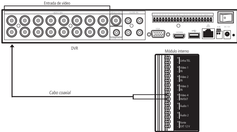
Gravar imagens do videoporteiro no DVR (Cabo coaxial)
