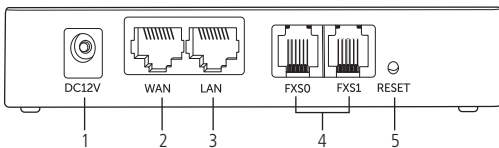
Visão posterior das conexões do ATA 200
