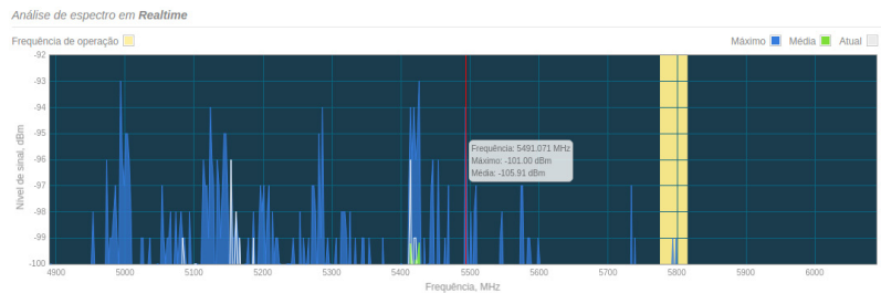
Análise de espectro – Nível de sinal, dBm
