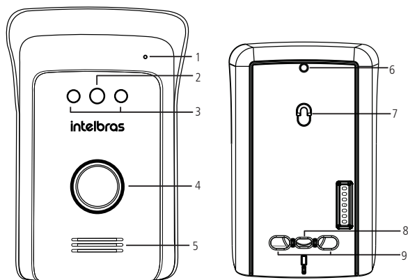
Módulo externo IVR 1010
