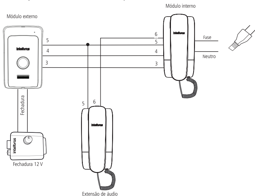
Exemplo de instalação do IPR 1010 com extensão de áudio e fechadura
