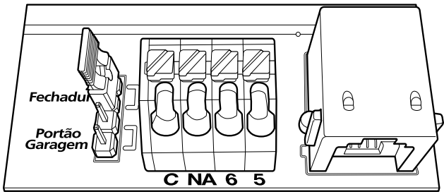
Jumpers e conectores
