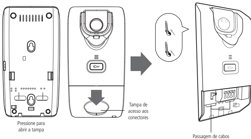
Fixação da extensão de áudio
