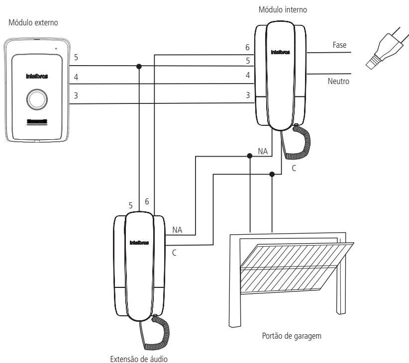
Exemplo de instalação do IPR 1010 com extensão de áudio e portão a motor
