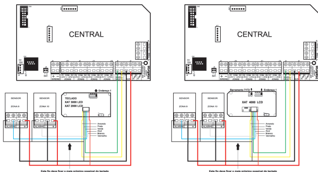
Esquema de ligação teclados linha XAT
