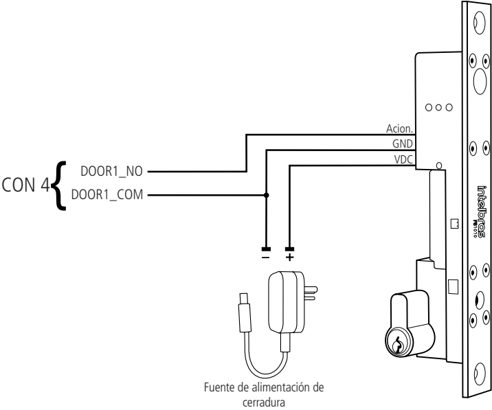
Ejemplo de conexión de cerradura de solenoide FS 1010
