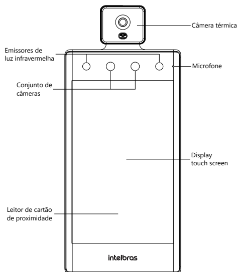
Visão frontal SS 7532 MF T W
