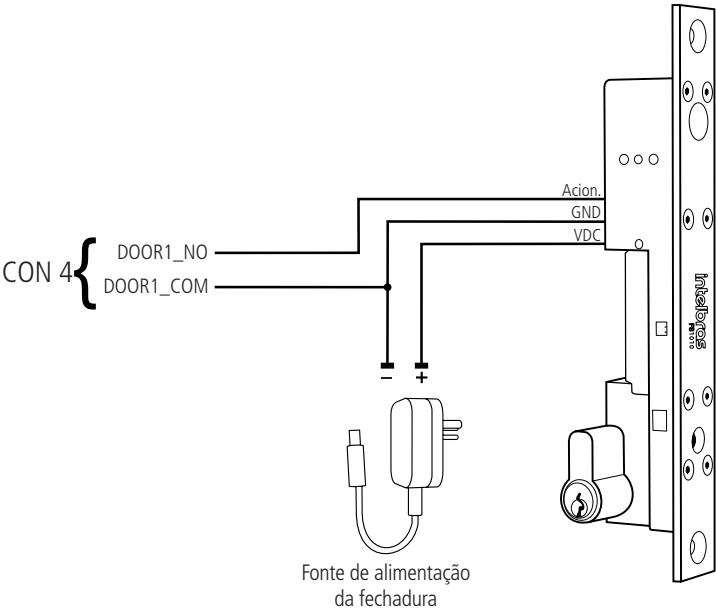
Exemplo de conexão de cerradura de solenoide FS 1010
