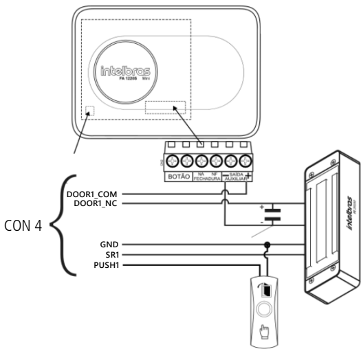
Ejemplo de conexión de cerradura electroimán con sensor
