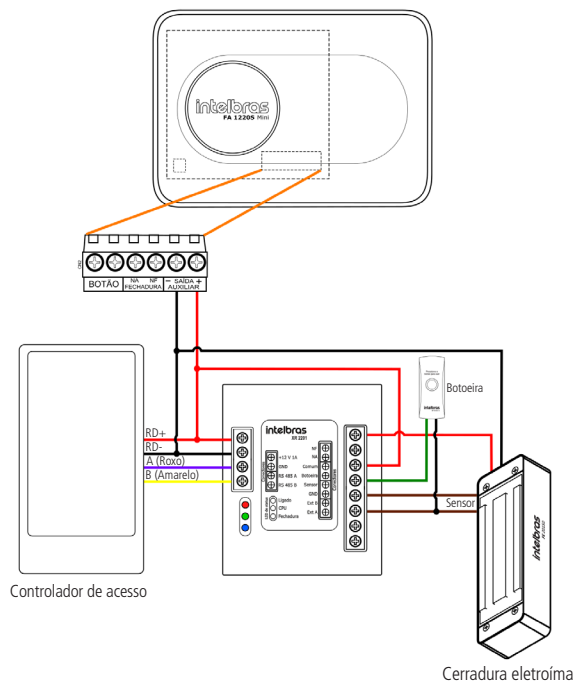
Diagrama de conexión con XR 2201
