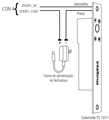
Exemplo de ligação de fechadura solenoide FS 1011
