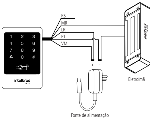
Ligação fechadura-eletrôimã
