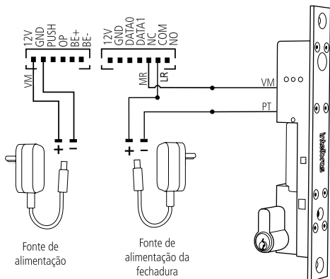
Fechadura solenóide FS 1011
