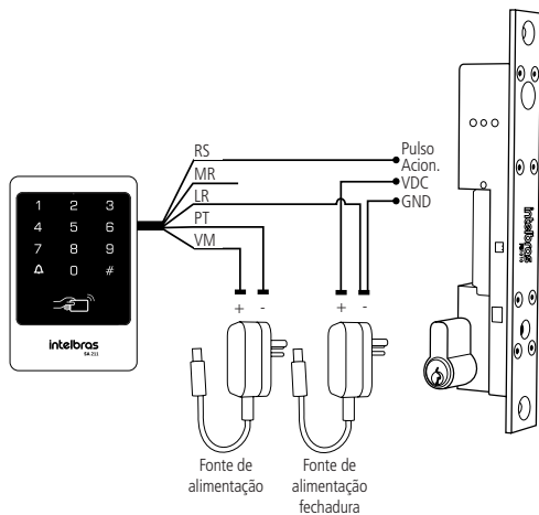
Ligação fechadura solenoide
