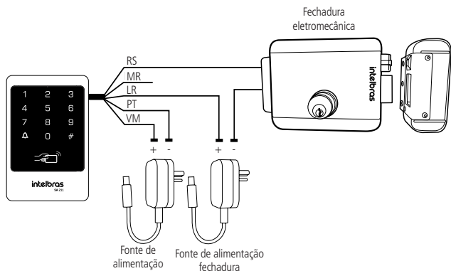
Ligação fechadura eletromecânica
