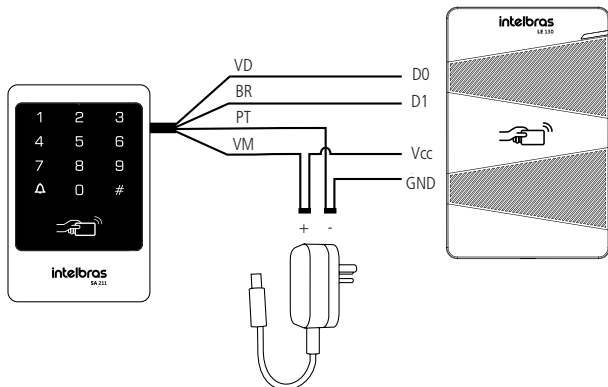
Fonte de alimentação
