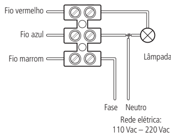
Conexões elétricas
