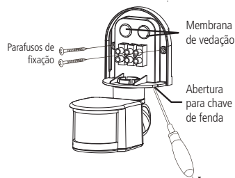
Fixação e instalação do sensor ESP 180 AE
