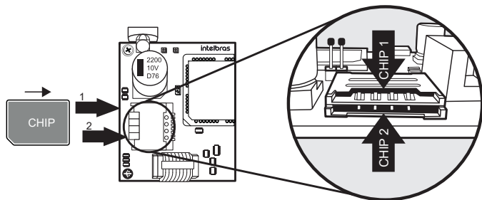
Asignación de chips en el módulo
