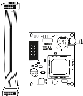
Módulo GPRS XAG 8000, módulo GSM XAG 8000 3G y módulo XG 4G
