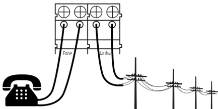
Esquema de conexión línea telefónica en el módulo FXO 8000.
