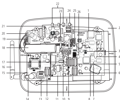
Central de alarma AMT 8000
