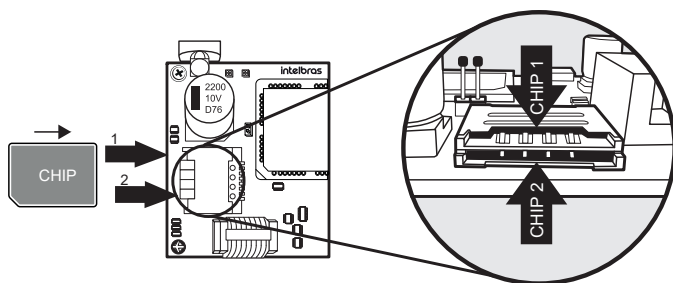
Colocación de chips en el módulo
