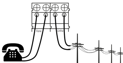
Esquema de ligação linha telefônica no módulo FXO 8000
