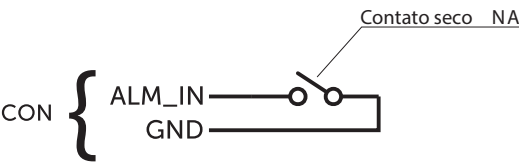
Ejemplo de conexión de entrada de alarma
