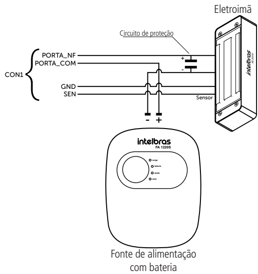
Exemplo de ligação de fechadura eletroimã
