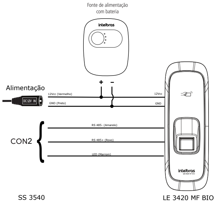
Exemplo ligação com LE 3420 MF BIO
