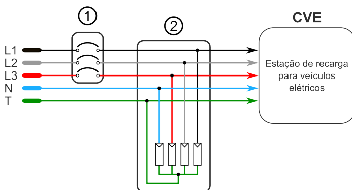
Quadro de proteções elétricas
