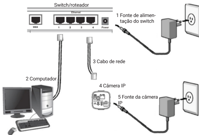
Conexão através de switch/roteador sem PoE
