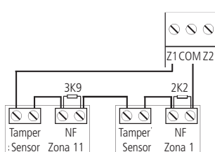
Ligação para sensores que possuem tamper
