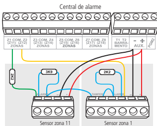
Ligação de sensor sem tamper
