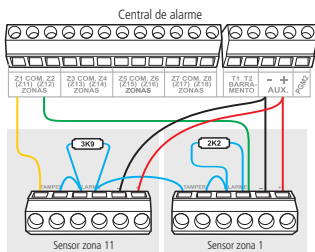
Ligação dos dois sensores com tamper
