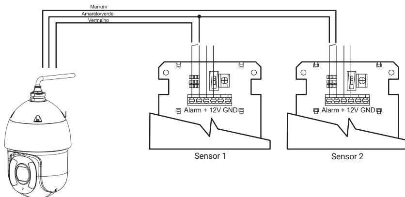
Conexão dos dispositivos de alarme
