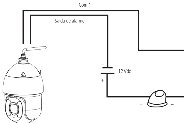
Conexão dos dispositivos de alarme
