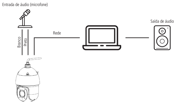
Conexão entrada de áudio da câmera
