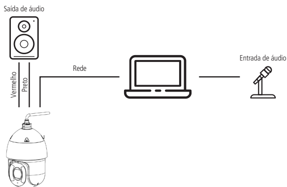
Conexão saída de áudio da câmera
