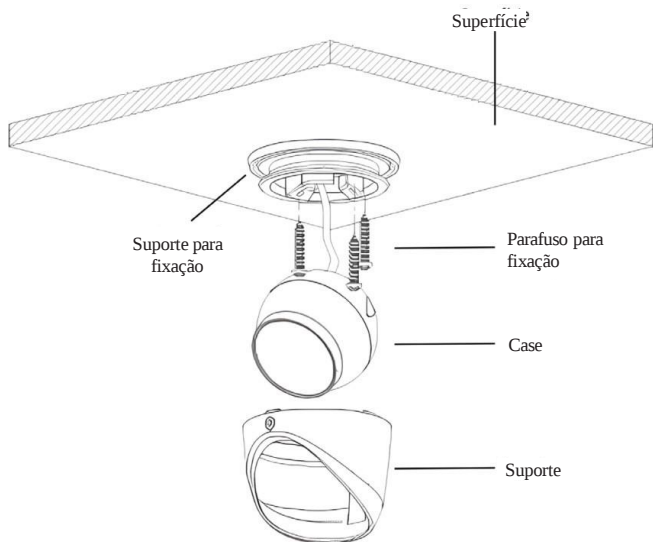
Vista detalhada VIPC 1230 D G2
