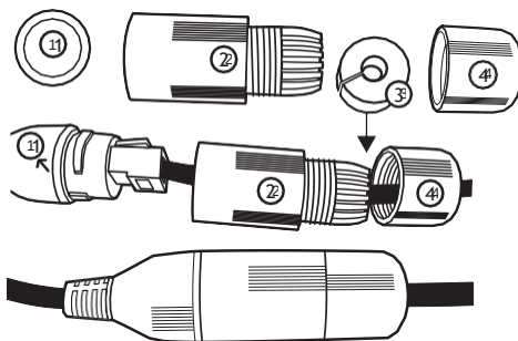
Conector de proteção
