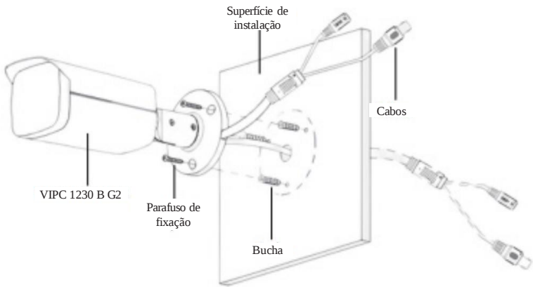
Vista detalhada VIPC 1230 B G2
