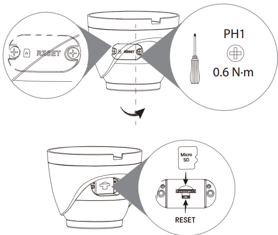
Acesso ao Botão de Reset e SD Card da VIPW 1430 D
