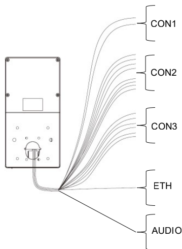
Visão traseira
