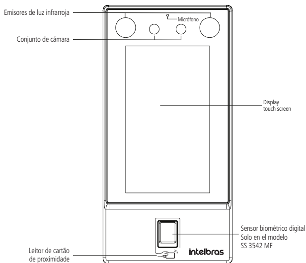
Visão frontal SS 3542 MF
