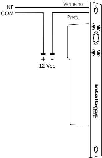
Solenóide FS 1011
