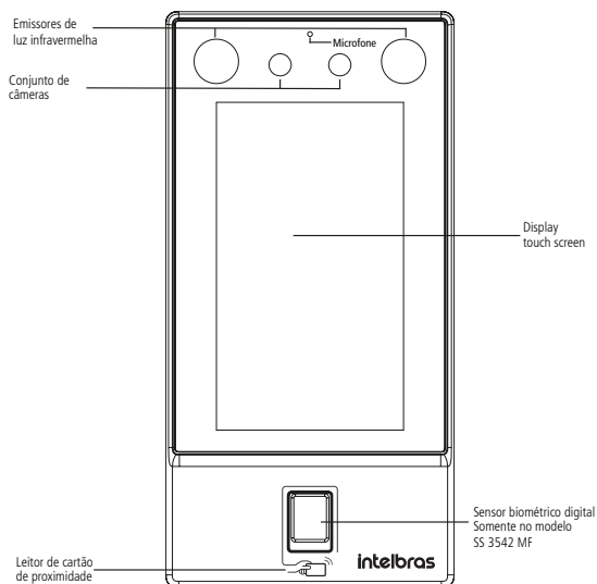
Visão frontal SS 3542 MF
