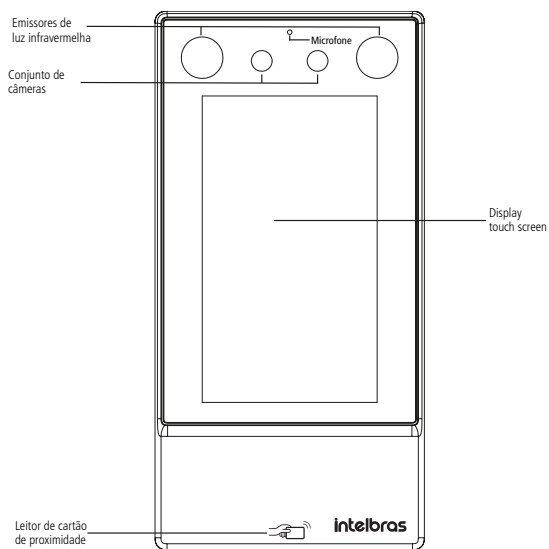
Visão frontal SS 3532 MF W
