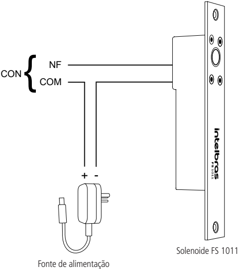
Exemplo de ligação de fechadura solenoide FS 1011
