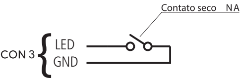
Exemplo de ligação de entrada de alarme
