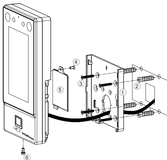
Modelo de fixação
