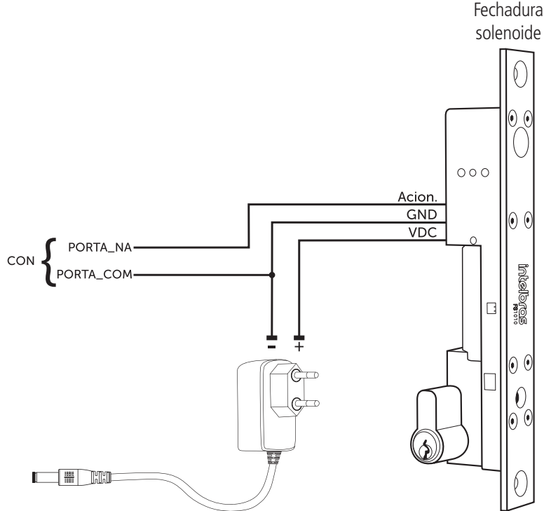
Exemplo de ligação de fechadura solenoide FS 1010
