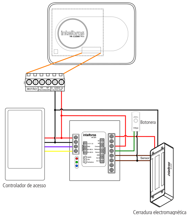
Esquema de ligación con XR 2201
