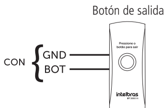
Ejemplo de conexión de botón de salida
