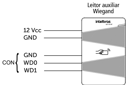
Exemplo de ligação de leitor Wiegand
