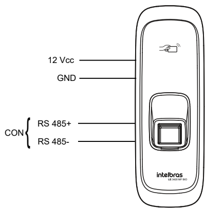
Ejemplo de conexión de lector biométrico digital
