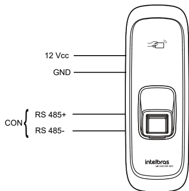
Exemplo de ligação de leitor biométrico digital
