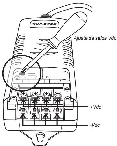
Visão frontal
