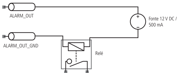
Esquema de saída de alarme VIP 5550 Z IA
