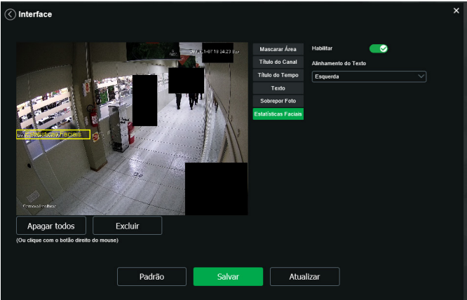
Estatísticas Faciais
