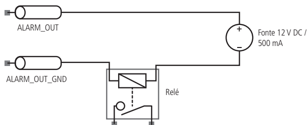
Esquema de saída de alarme VIP 5550 DZ IA
