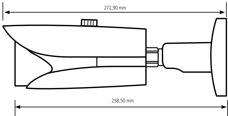
Visão lateral VIP 5550 Z IA
