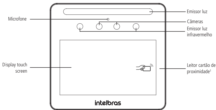
Vista frontal SS 3530 MF FACE W ou SS 3530 MF FACE
