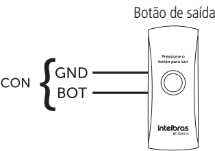
Exemplo de ligação de botão de saída
