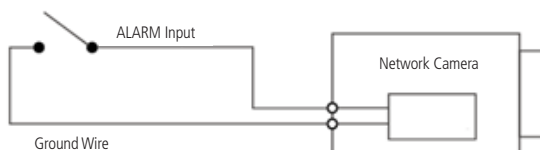
Esquema de entrada de alarme VIP 5550 Z IA
