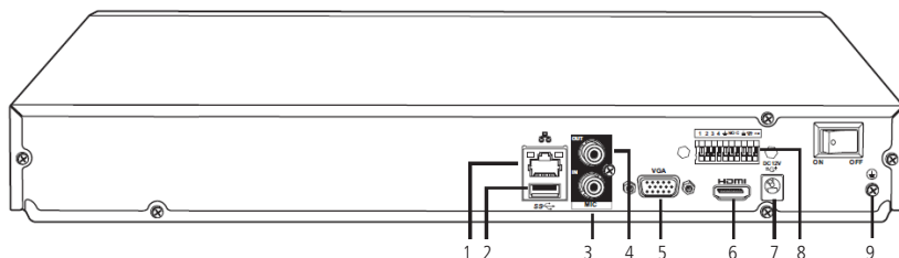
Painel posterior
