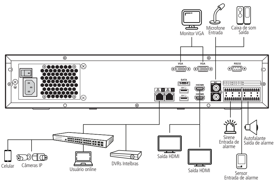
Exemplo de conexão - NVD 5124
