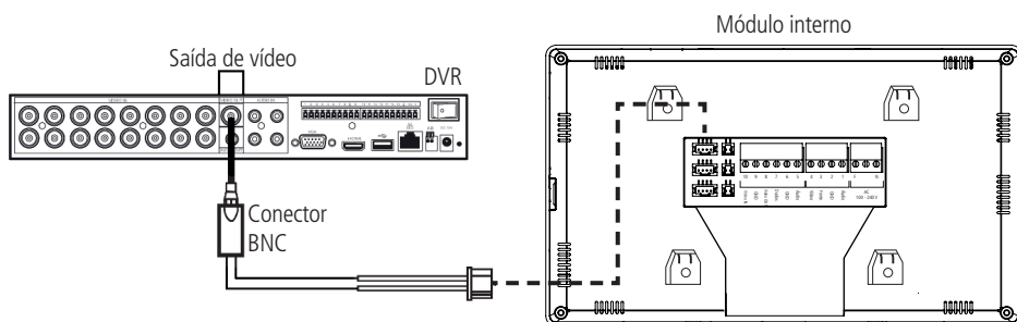
Saída de vídeo do DVR com monitor
