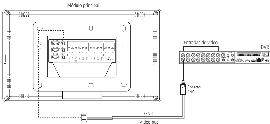
Instalação da saída de vídeo do monitor no DVR
