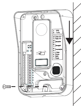
Fixação do segundo parafuso (inferior) da 4x2
