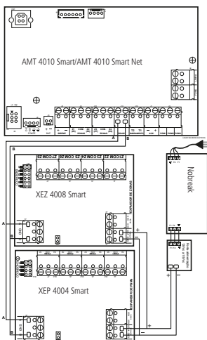
Esquema de ligação módulos de expansão
