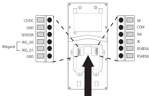
Conexão Ethernet RJ45 - 10/100
