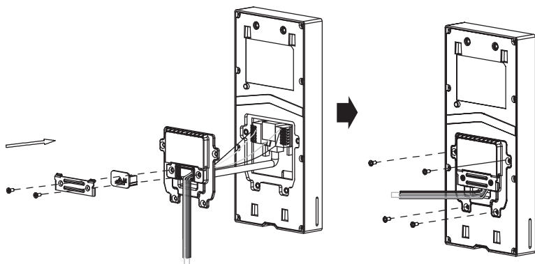
Conhecendo a sequência de montagem
