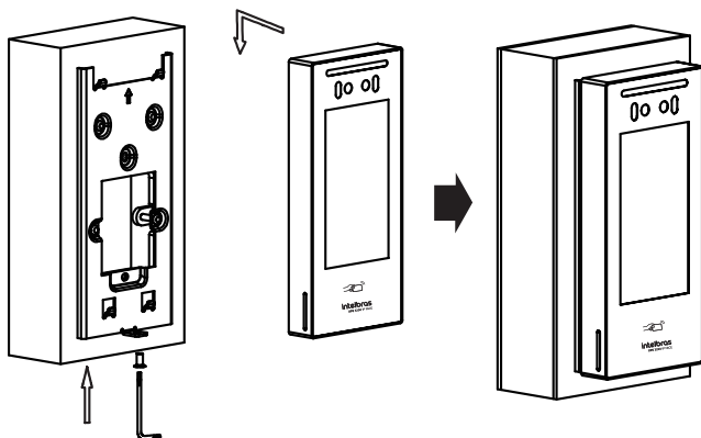
Conhecendo a sequência de montagem
