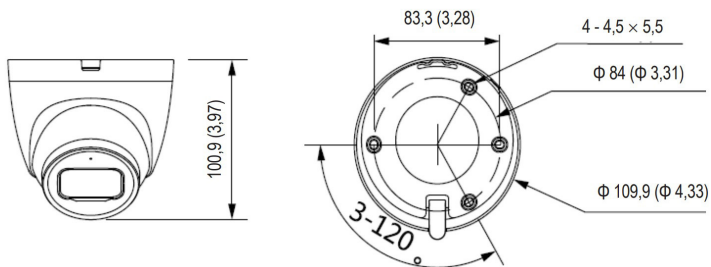
VIP 3220 D FC IA
