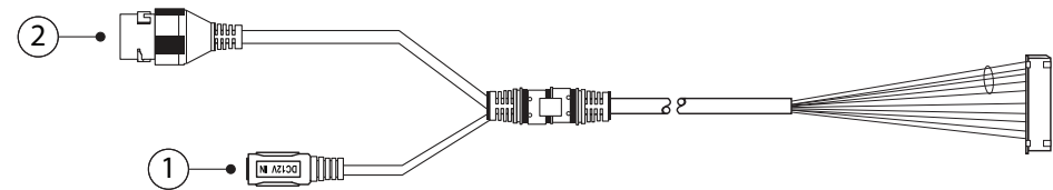
Cabo multifunções VIP 3220 FC IA e VIP 3220 D FC IA
