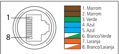
Cabo multifunções VIP 3220 D FC IA
