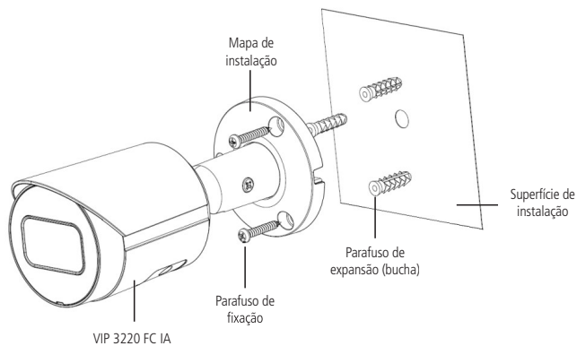
Vista detalhada VIP 3220 FC IA
