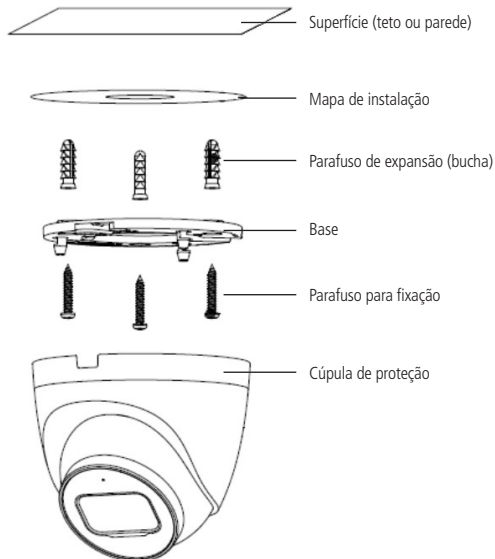
Vista detalhada VIP 3220 D FC IA
