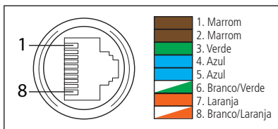
Cabo multifunções VIP 3230 B SL e VIP 3230 D SL
