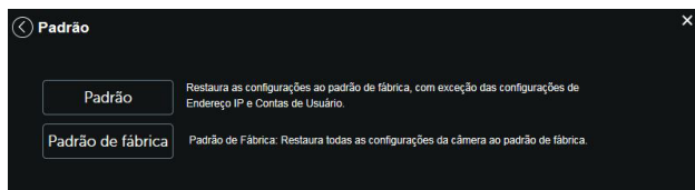
Configuração padrão
