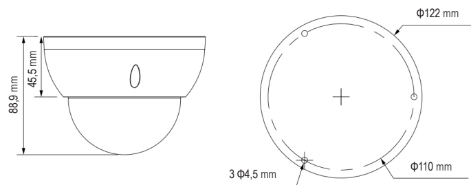
Visão lateral e frontal
