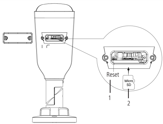
Visão Inferior
