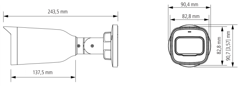
Visão lateral e frontal
