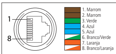
Cabo multifunções VIP 3240 Z G2
