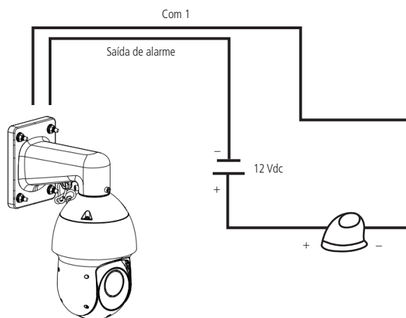
Conexão dos dispositivos de alarme
