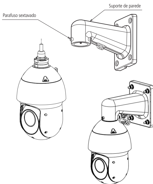
Instalação do suporte
