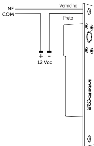
Solenoido FS 1011
